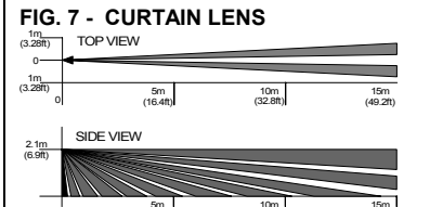
FIG. 7 - CURTAIN LENS
